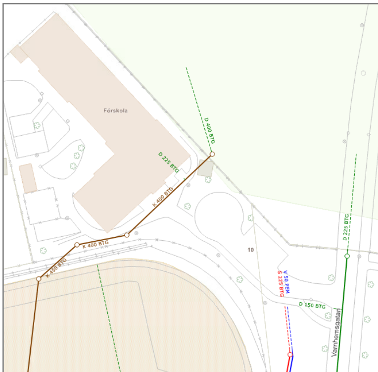
Ledningsnätskarta
